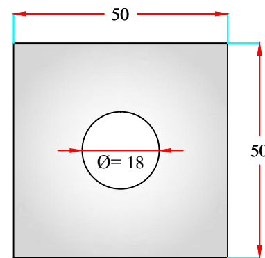
واشر مربعی با ابعاد ۵۰x۵۰x۳ میلیمتر
